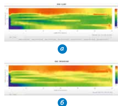
Рис. 2. Пример карт с уровнем загазованности \text{CO}_2 (а) и температурного поля птичника (б)
