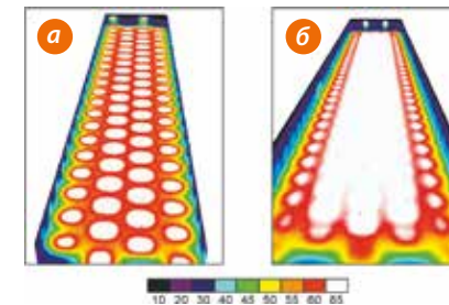
Рис. 2. Светотехнический расчет для птичника напольного содержания цыплят-бройлеров с освещенностью 60 лк, оборудованного на высоте 3 метра 84 светодиодными светильниками CH500-12-26-T мощностью 12 Вт (а) и 165 светильниками CH300-6-13-T на 6 Вт (б) для 4 и 5 линий освещения соответственно
